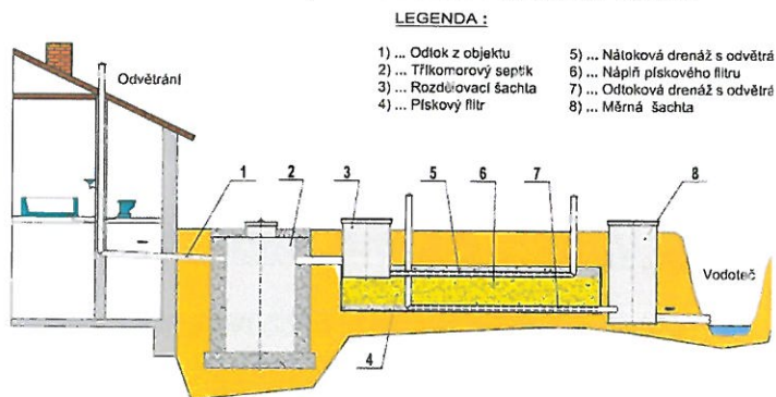
Schéma víceetapňové ČOV septik + pískový filtr
